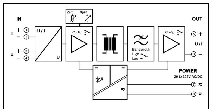
Prinzipschaltbild
